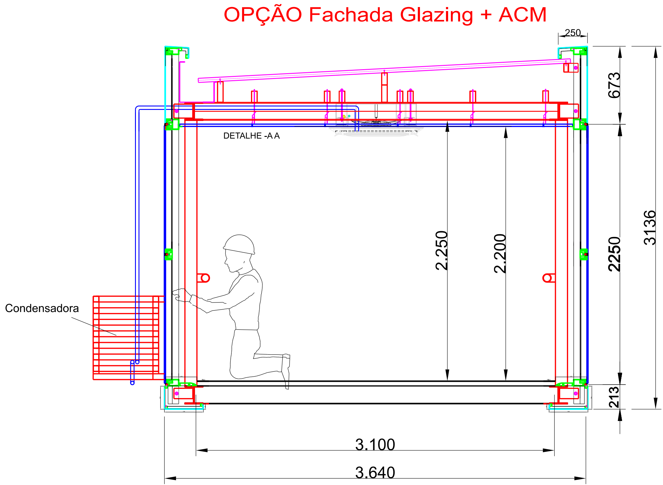
CORTE - AA ESC: 1:20
