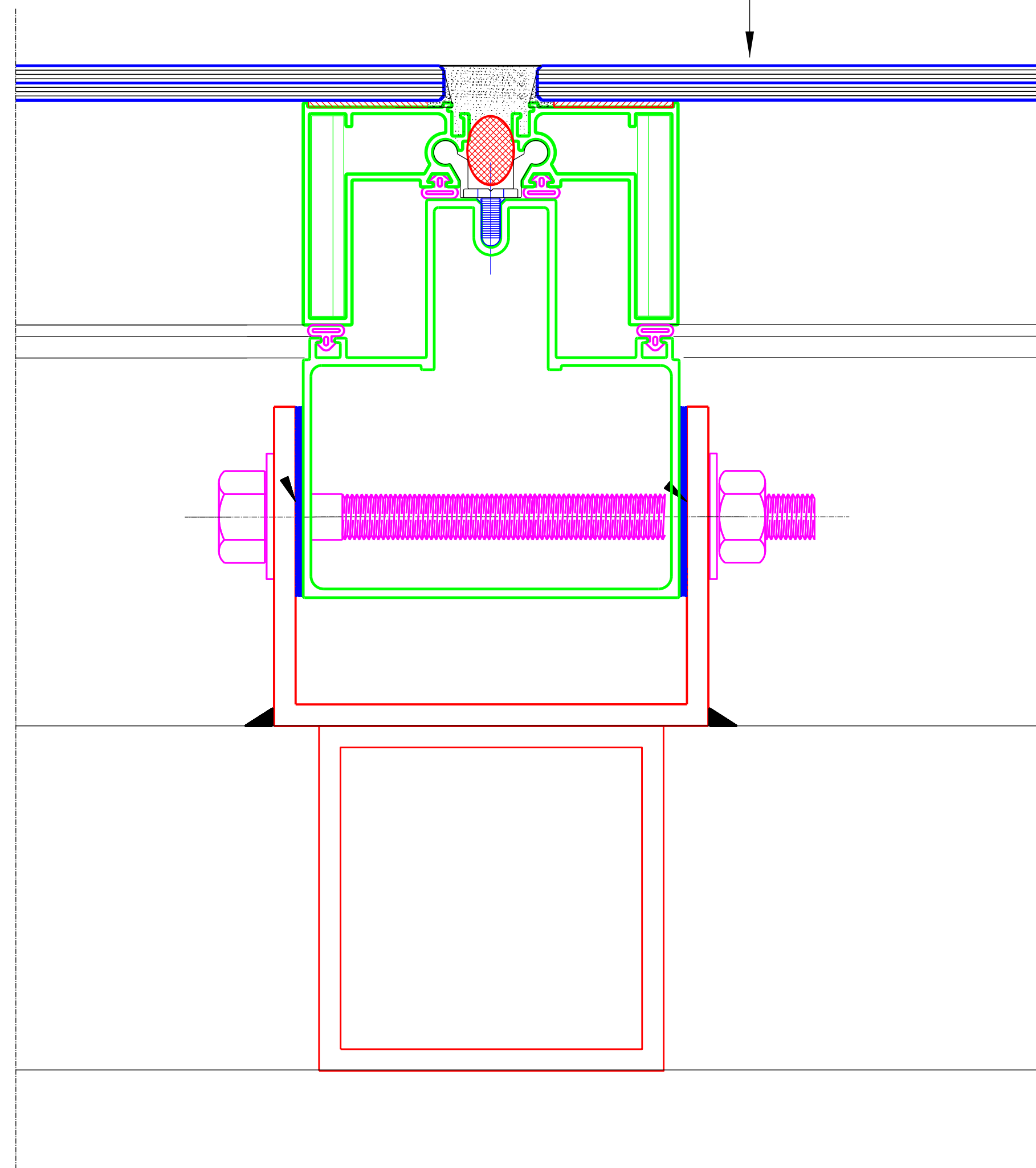
DETALHE -D
